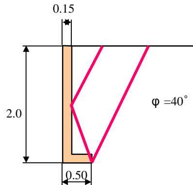
(b) 改良試行くさび法による解析
