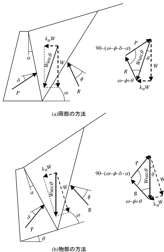
図 10 震度法による地震時土圧
