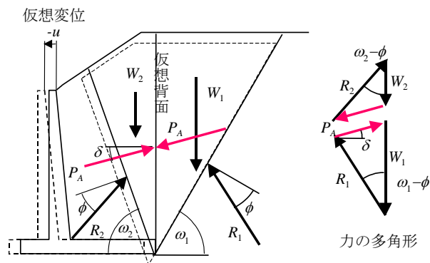
図9 改良試行くさび法
