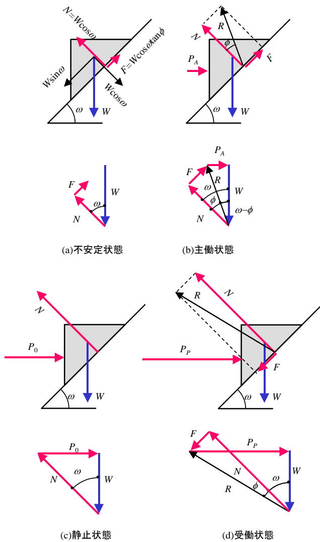
図3 斜面上の剛体ブロックの安定問題
