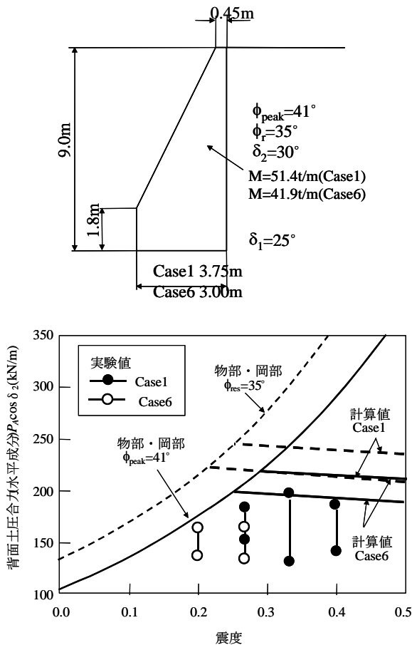
図 12 建設省土木研究所による動的遠心模型実験 10)
