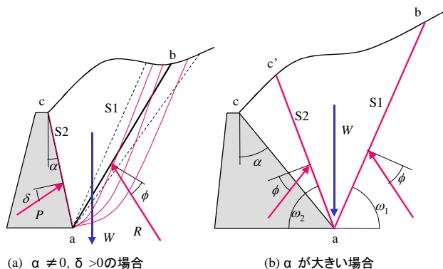
図6 主働すべり面
