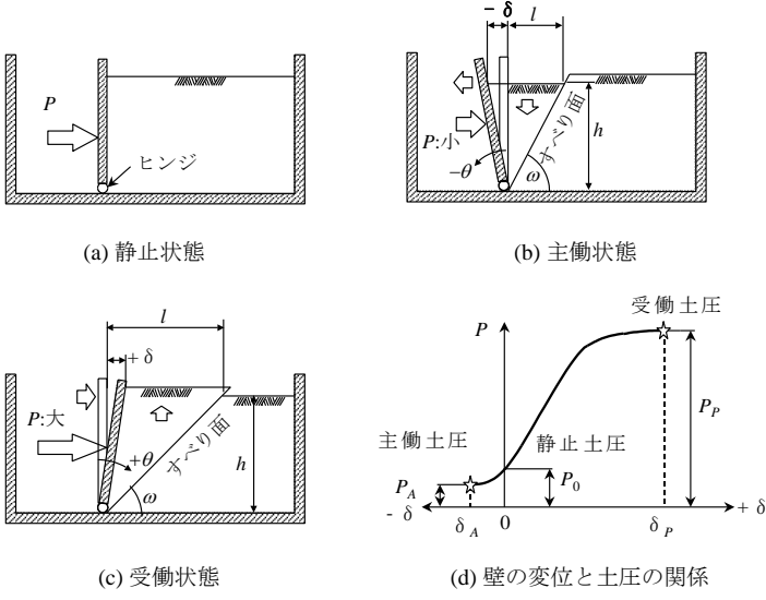
図2 壁の変位と土圧 4)
