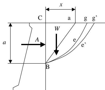
図1 クーロンの土圧理論 1)
