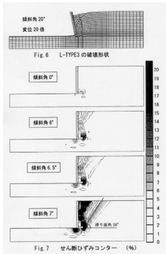
(a) FEMによる解析(田中・今田)
