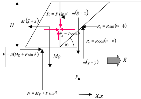
図 11 動土圧の解析モデル
